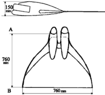
Monopalet Ölçüleri
